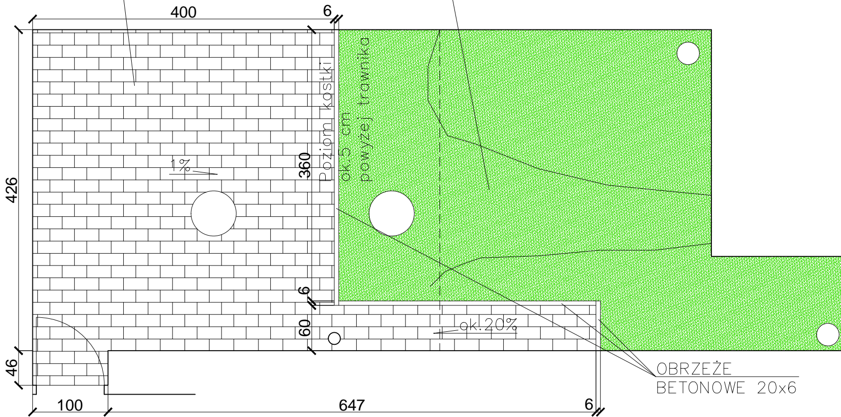
RYS. 2 RZUT NAWIERZCHNI - STAN PROJEKTOWANY
